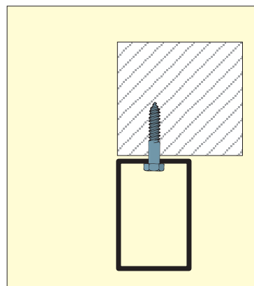
6. PK6 Square steel/alu 40x60 mm
